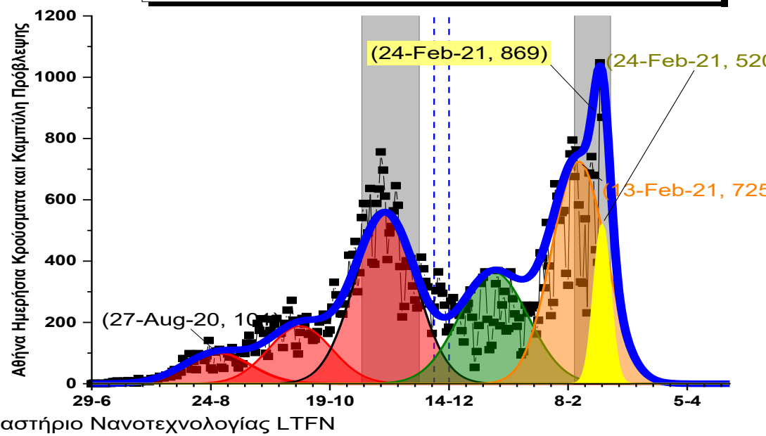
Αθήνα Ημερήσια Κρούσματα και Καμπύλη Πρόβλεψης
